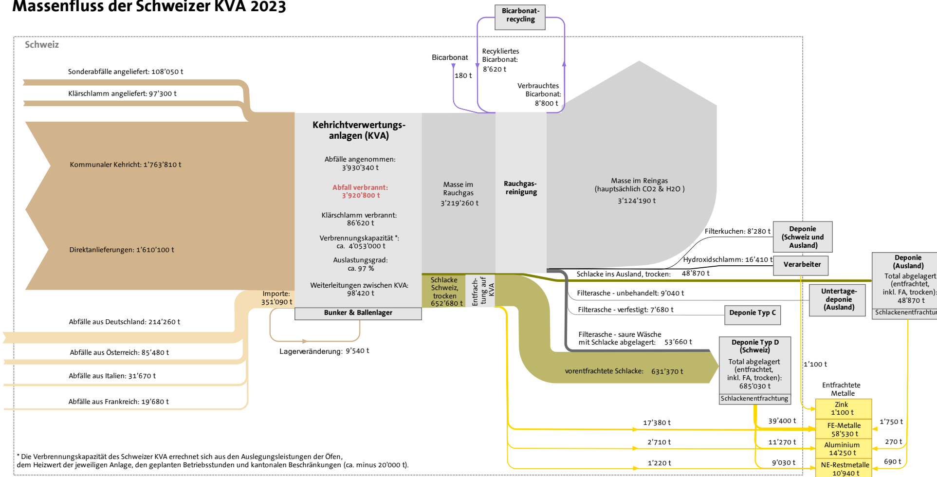
Abbildung 19: Massenflussdiagramm 2023
