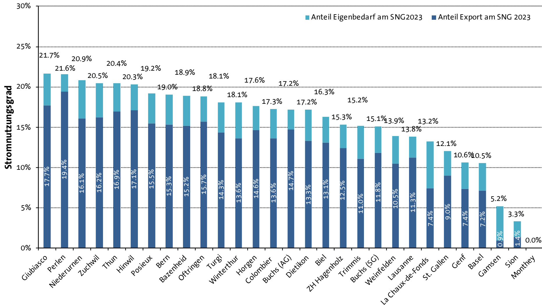
Abbildung 17: Stromnutzungsgrad 2023
