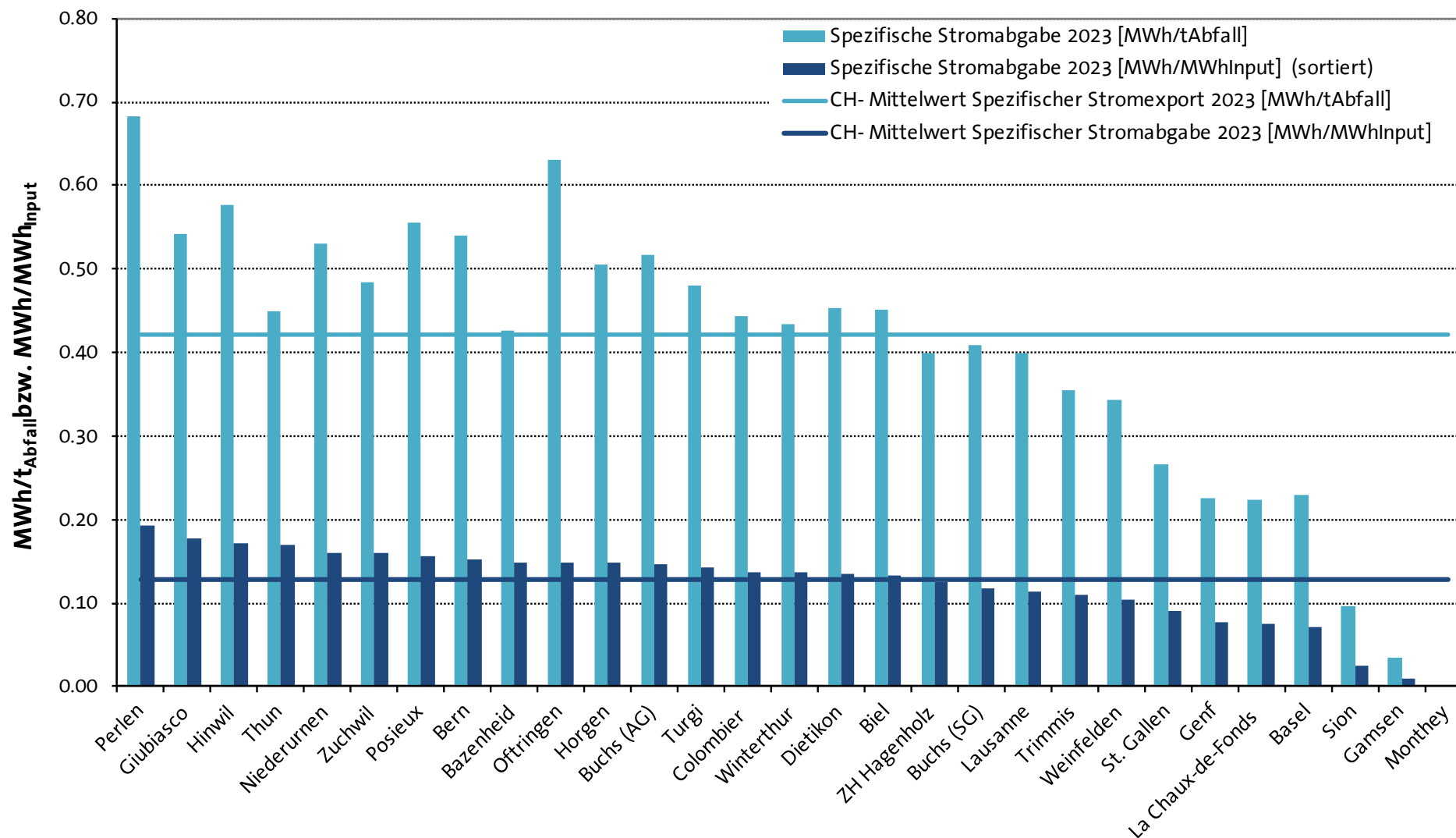
Abbildung 14: Spezifischer Stromexport 2023
