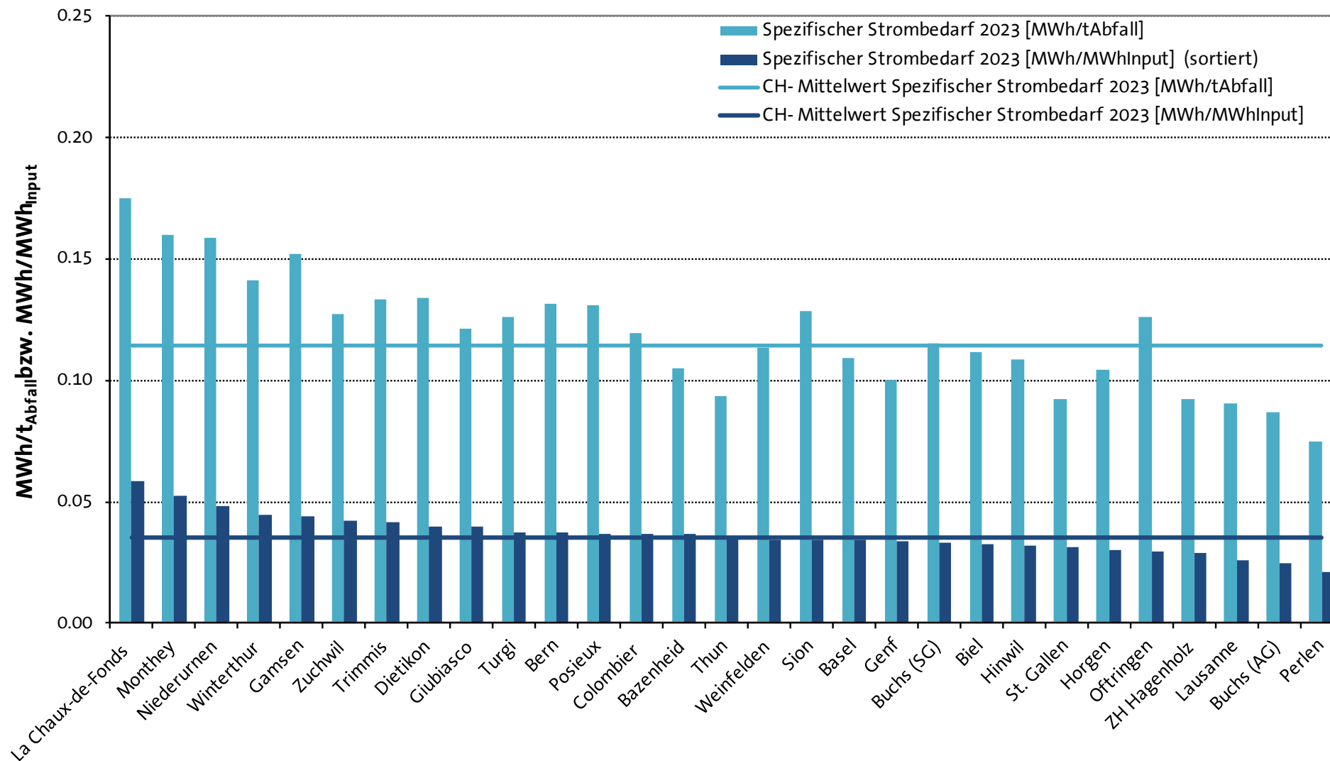
Abbildung 15: Spezifischer Stromeigenbedarf 2023
