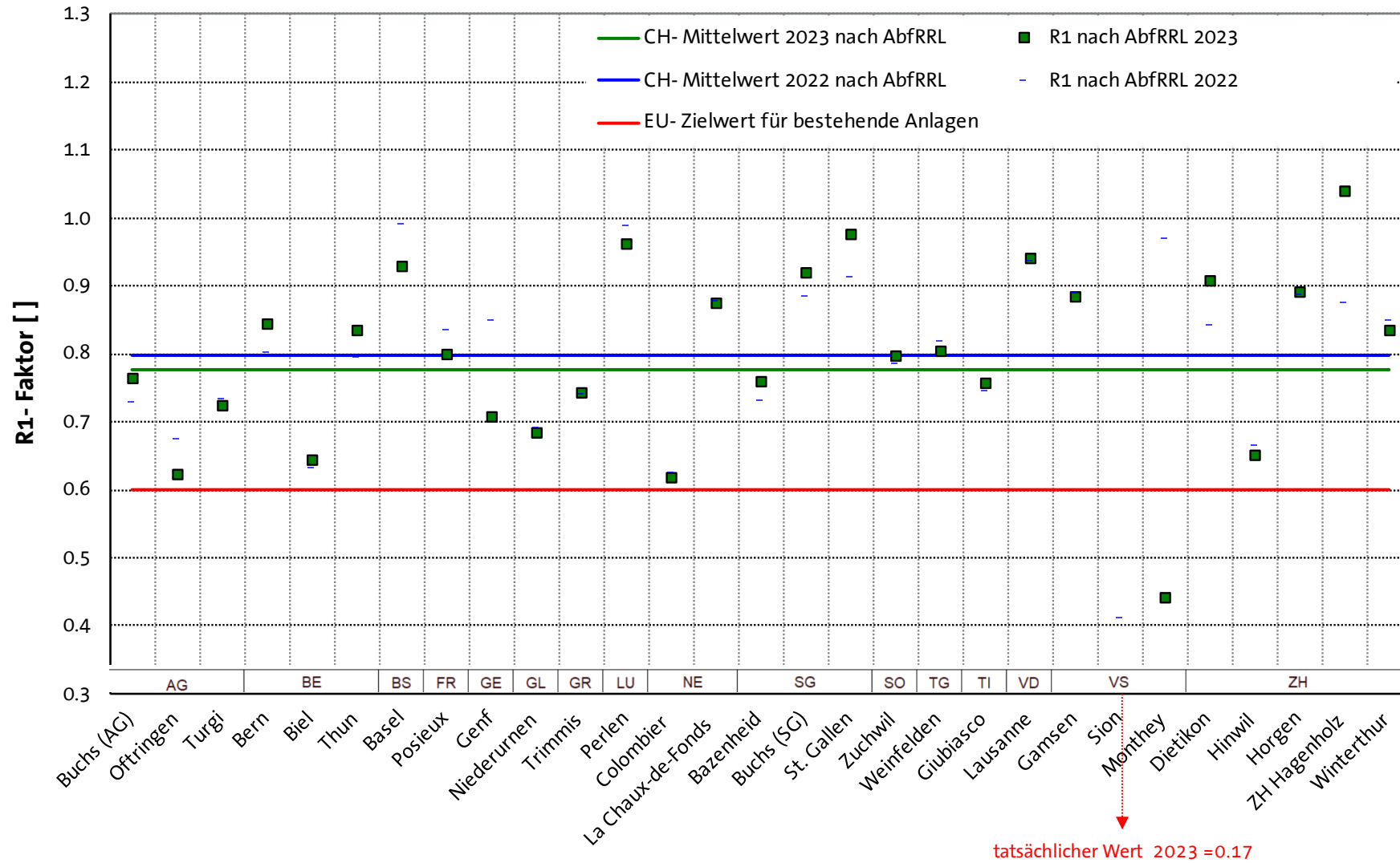
Abbildung 8: R1-Faktor 2023 und 2022
