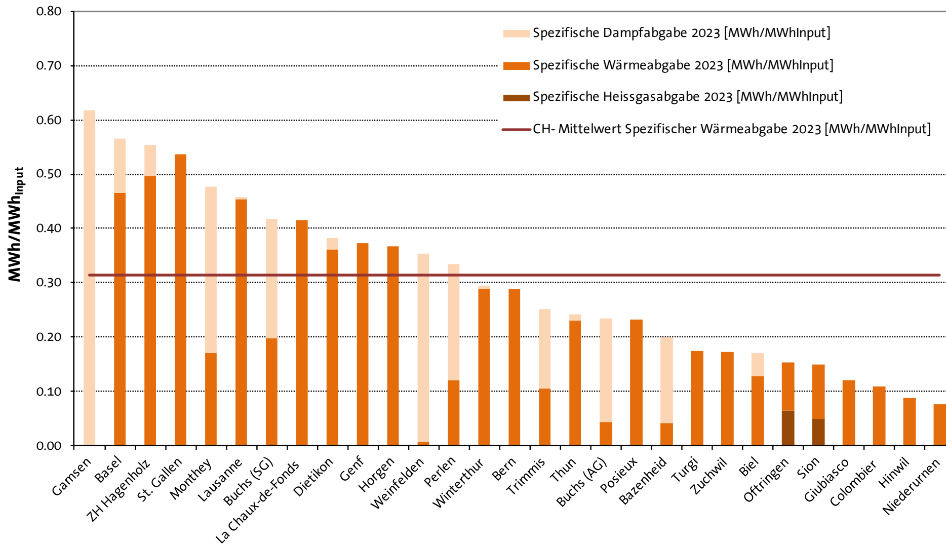
Abbildung 12: Spezifischer Wärmeexport pro Energieinput 2023
