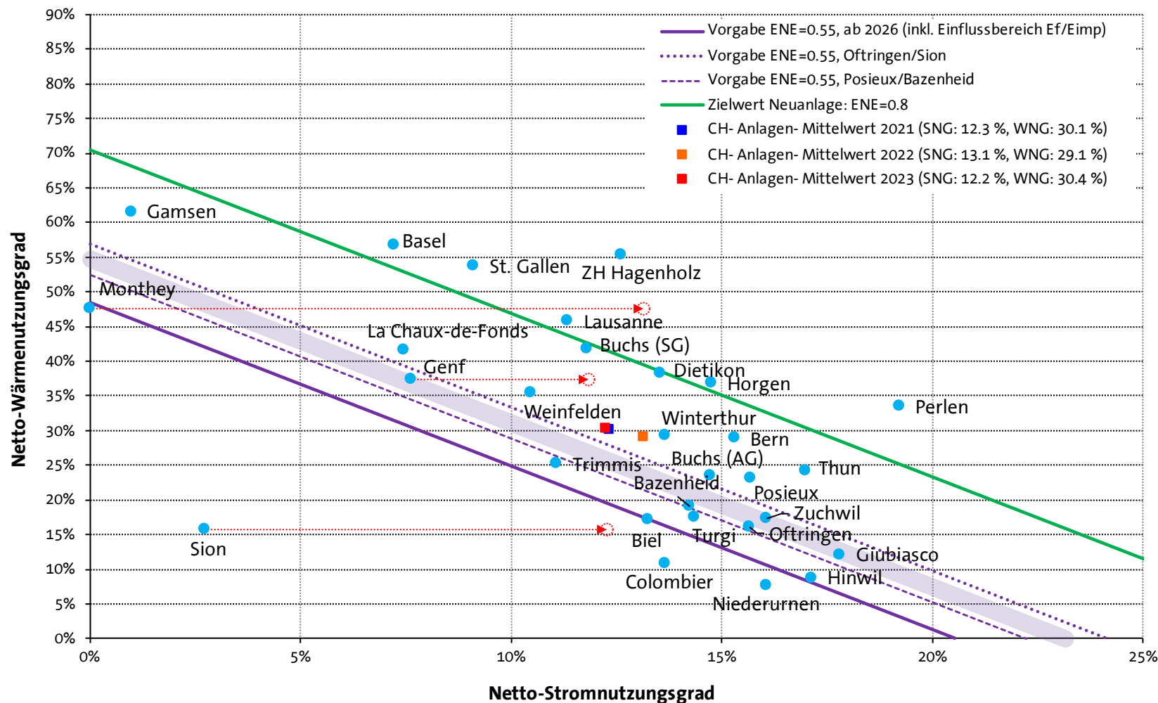
Abbildung 6: Energetische Nettoeffizienz ENE 2023 und Auswirkung durch Sonderzustände wie z. B. Turbinen- und Generatorausfall oder ausserplanmässigen Stillstand (rote Kreise und Pfeile)
