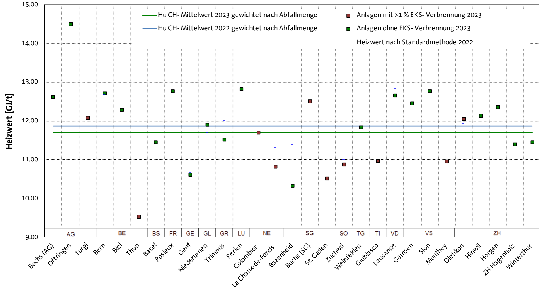
Abbildung 7: Heizwert 2023 und 2022
