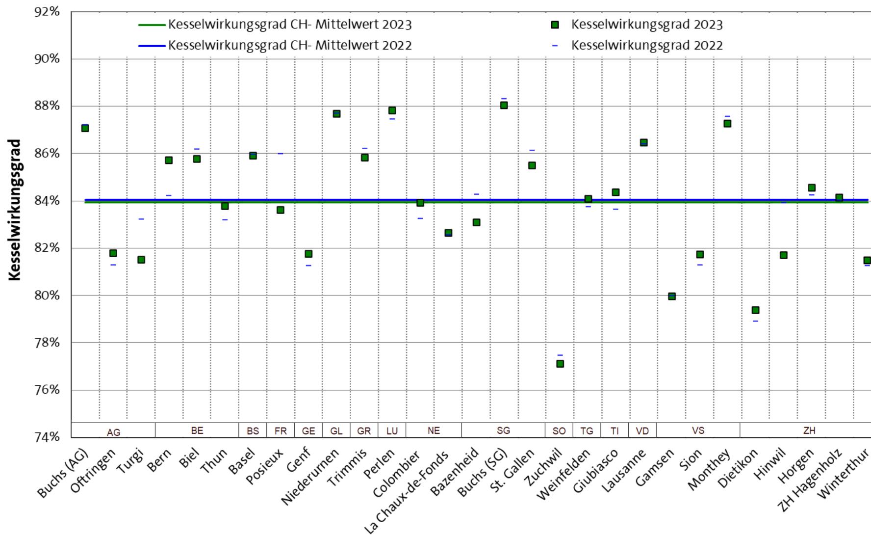
Abbildung 10: Kesselwirkungsgrad 2023 und 2022
