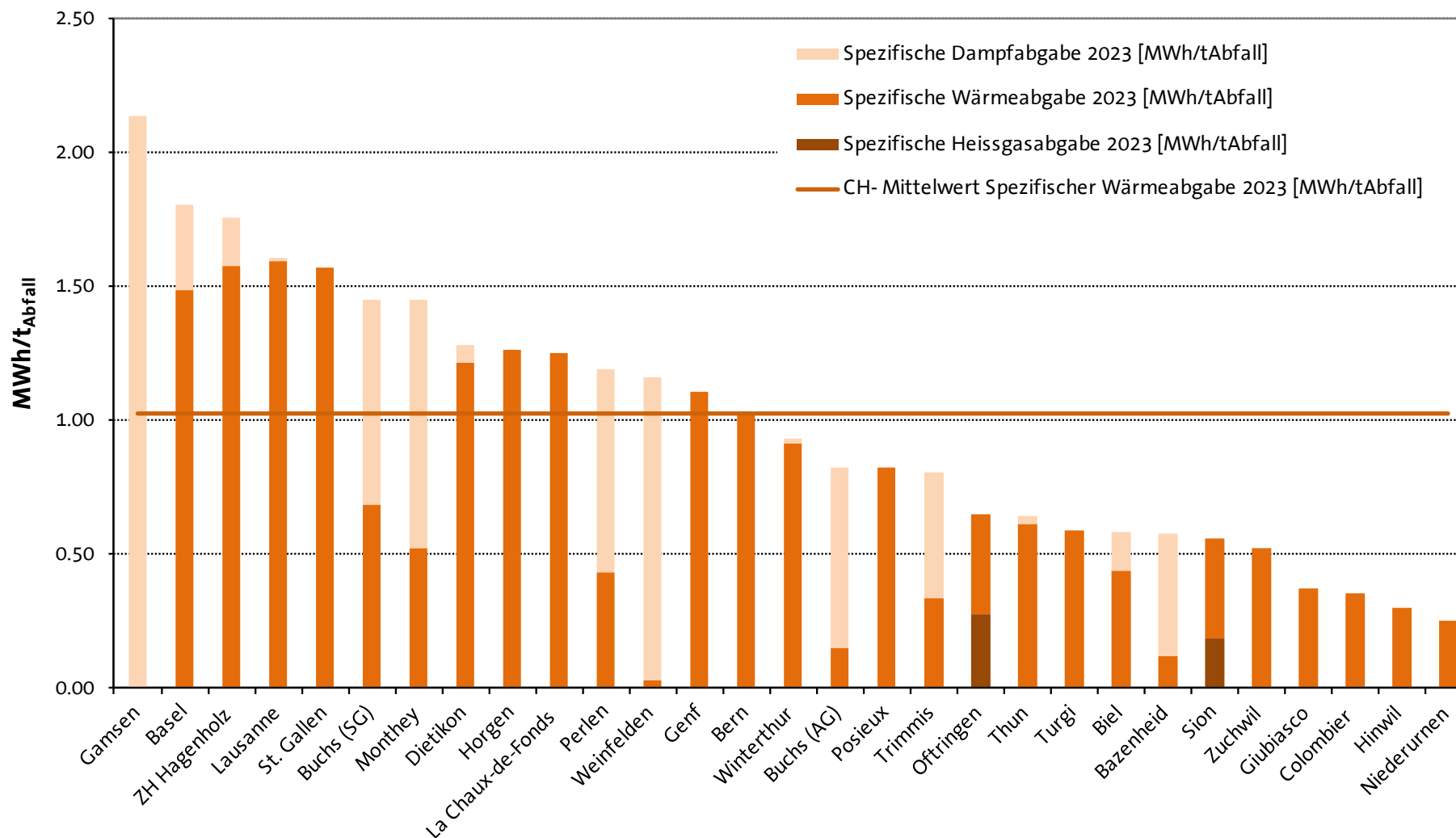
Abbildung 11: Spezifischer Wärmeexport pro Tonne Abfall 2023
