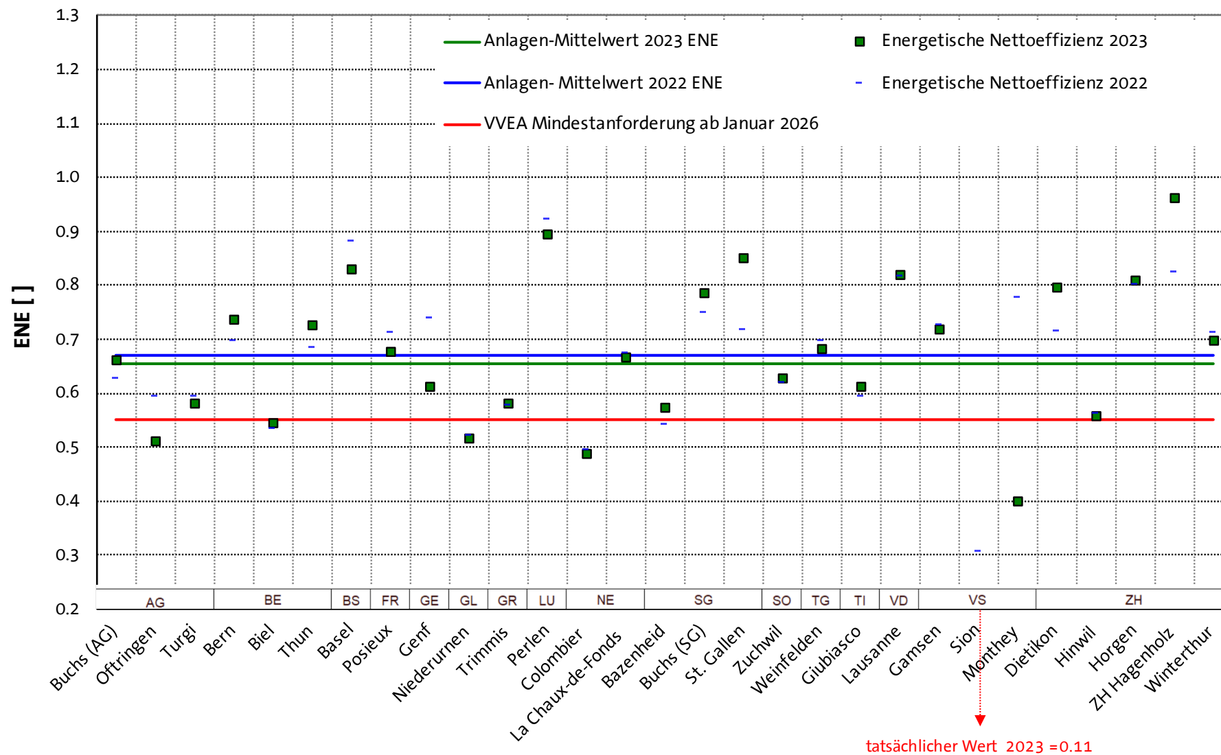
Abbildung 9: Energetische Nettoeffizienz ENE 2023 und 2022
