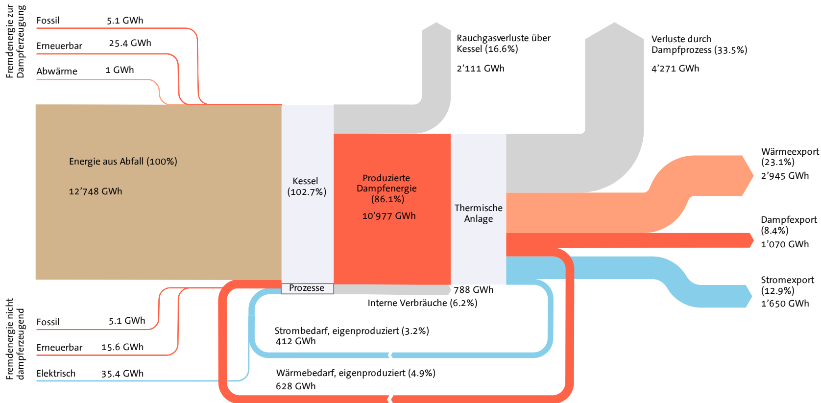
Abbildung 18: Energieflussdiagramm CH-KVA 2023
