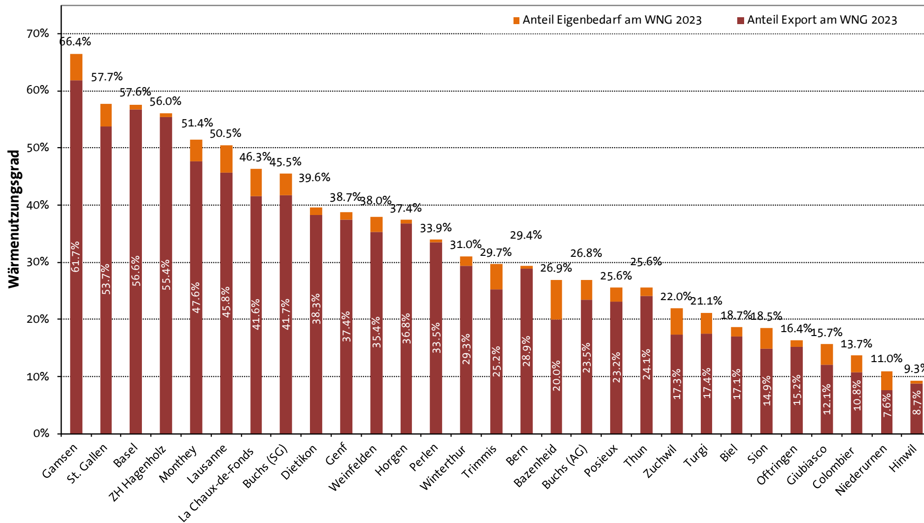
Abbildung 16: Wärmenutzungsgrad 2023
