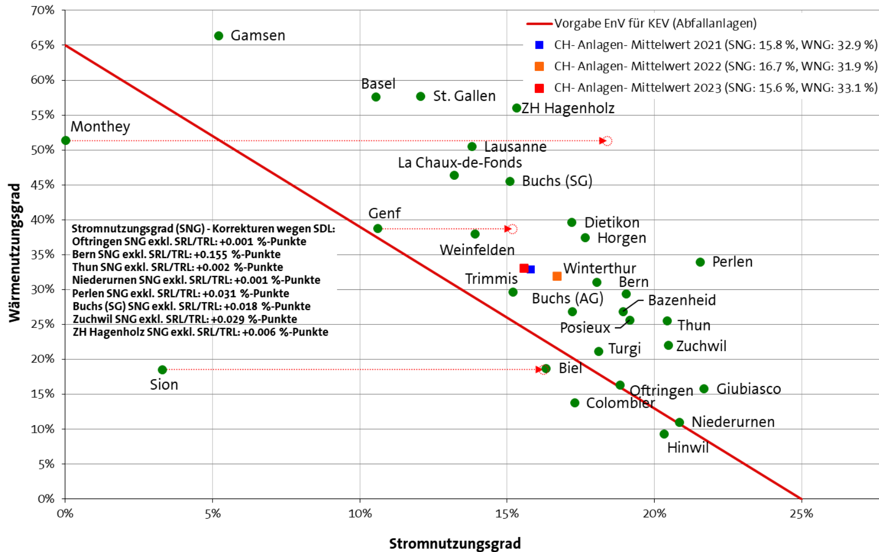
Abbildung 5: Energienutzungsgrad nach EnV, 2023 und Auswirkung durch Sonderzustände wie z. B. Turbinen- und Generatorausfall oder ausserplanmässigen Stillstand (rote Kreise und Pfeile)
