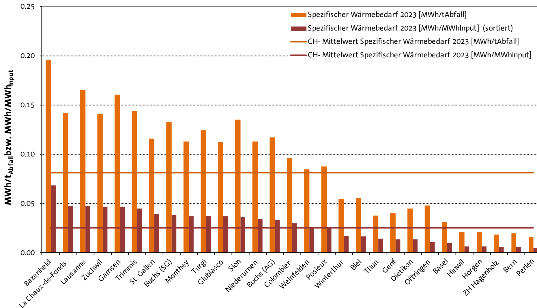
Abbildung 13: Spezifischer Wärmeeigenbedarf 2023
